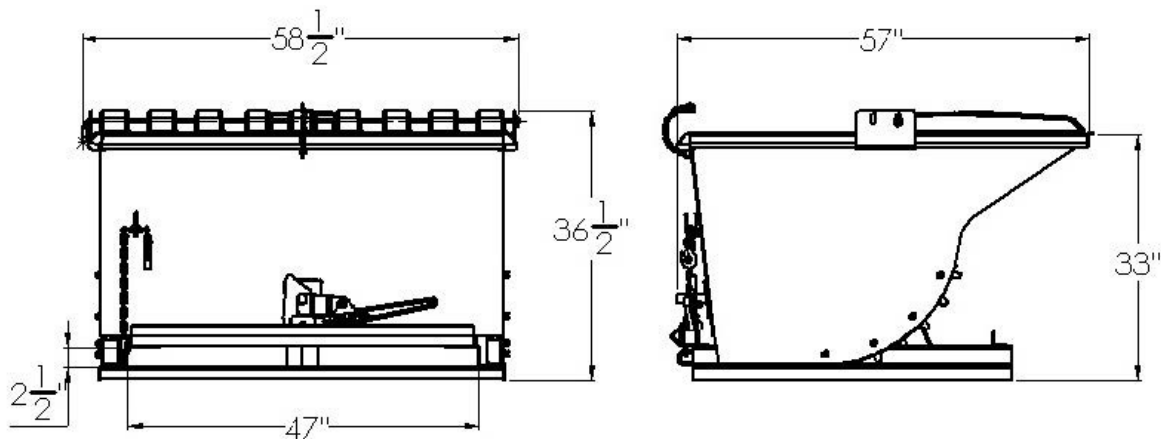
H-PLDB-270
